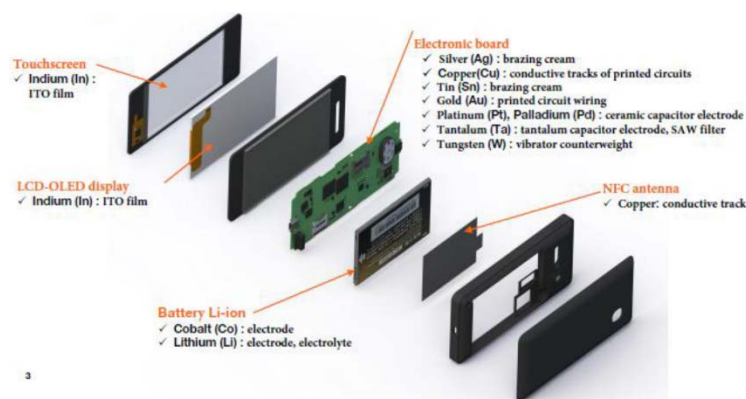
Illustration 12 : Composants de matériel informatique à l'exemple du smartphone
